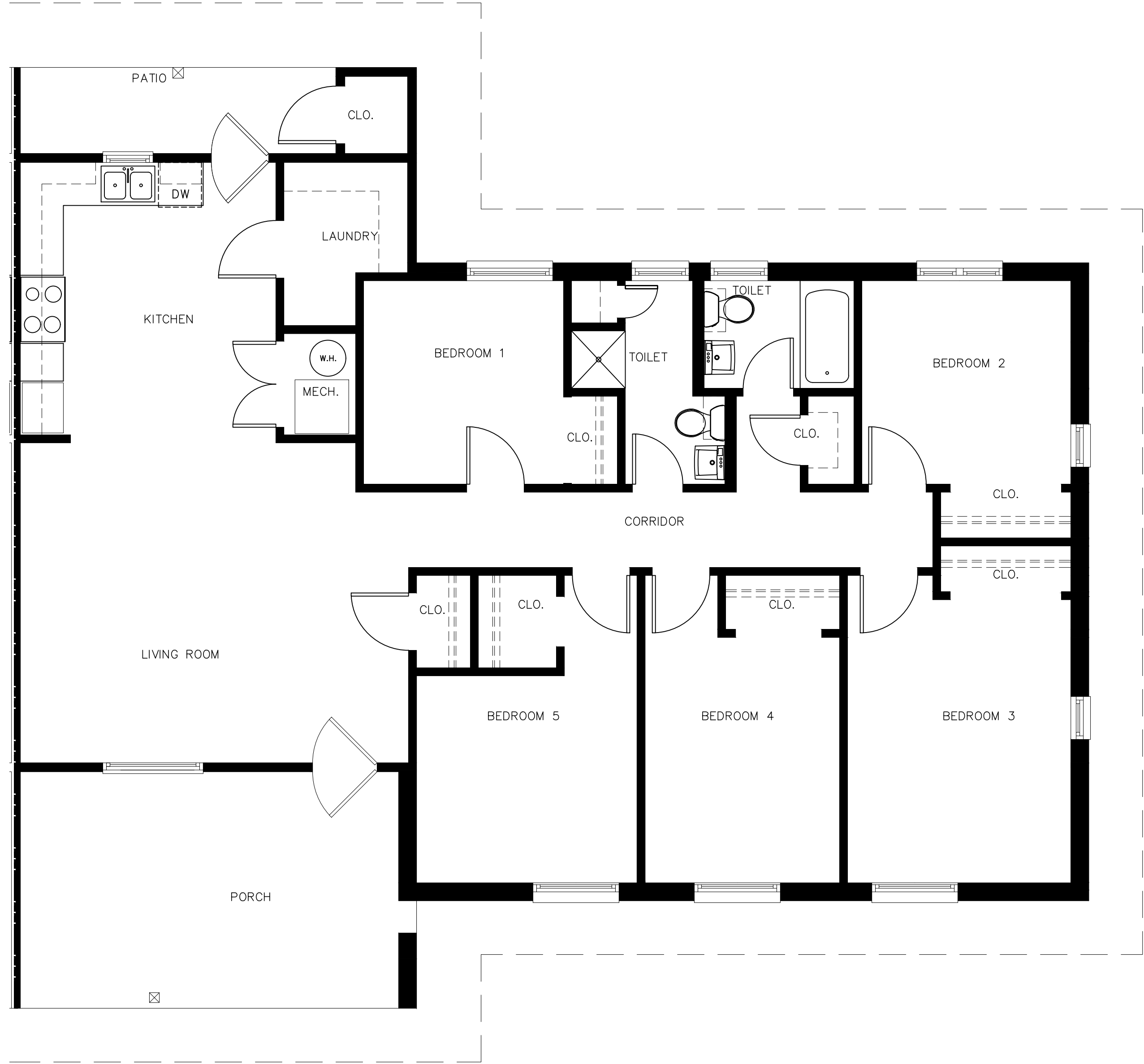
A 5 BEDROOM TYPE K SCALE: 1/4" = 1'-0"
