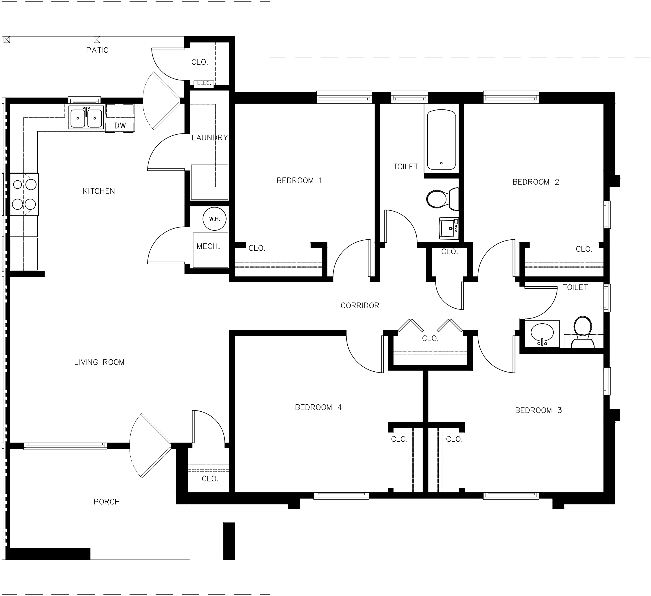
A 4 BEDROOM TYPE H SCALE: 1/4" = 1'-0"
